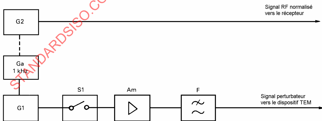
Figure 7 – Circuit de mesure pour l'immunité aux champs ambiants des récepteurs de radiodiffusion sonore
