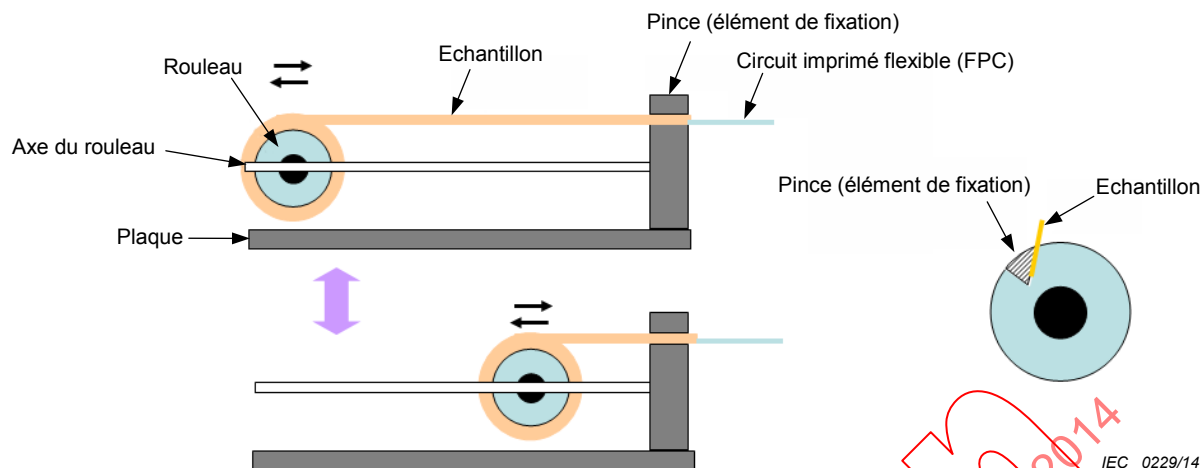
Figure 4 – Appareillage d'essai d'enroulement
