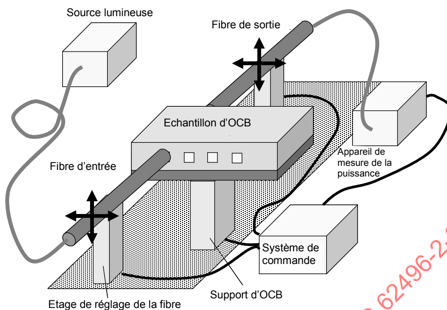
Figure 4 – Exemple de système de réglage de la position optique relatif à l'OCB de type E/S en extrémité
