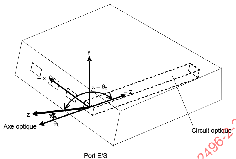
Figure 7 – Angle de défaut d'alignement des ports E/S dans un OCB de type E/S en extrémité
