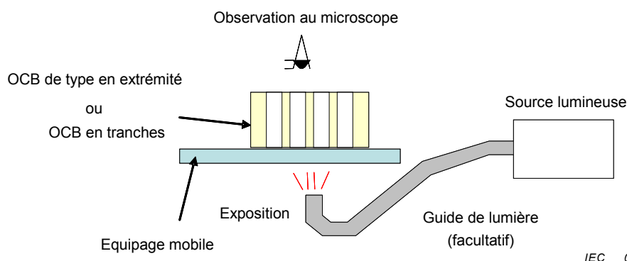
Figure 2 – Exemple de montage d'échantillon pour l'observation de la forme du cœur (OCB de type E/S en extrémité ou échantillon découpé en tranches)
