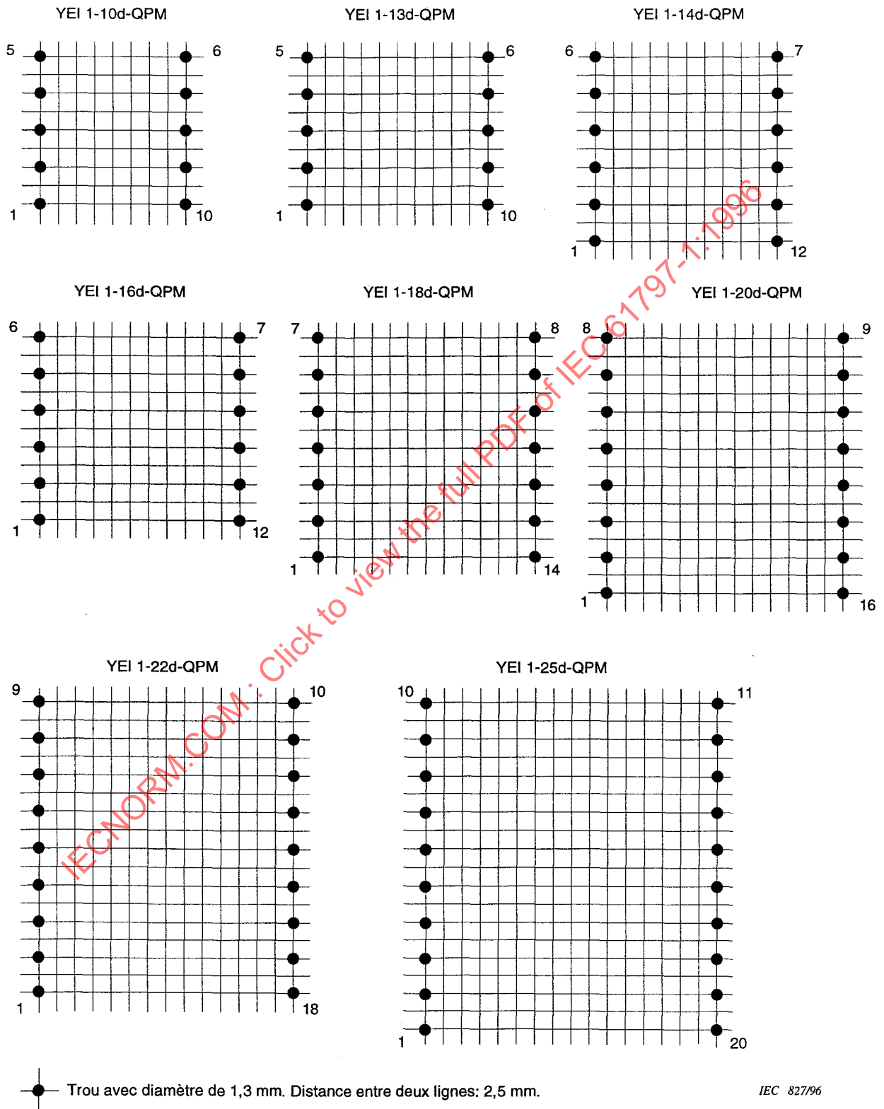
Figure 8 – Plans de grille pour carcasses de type YEI 1 pour montage sur carte à câblage imprimé, mode de montage à plat, plan de grille métrique
