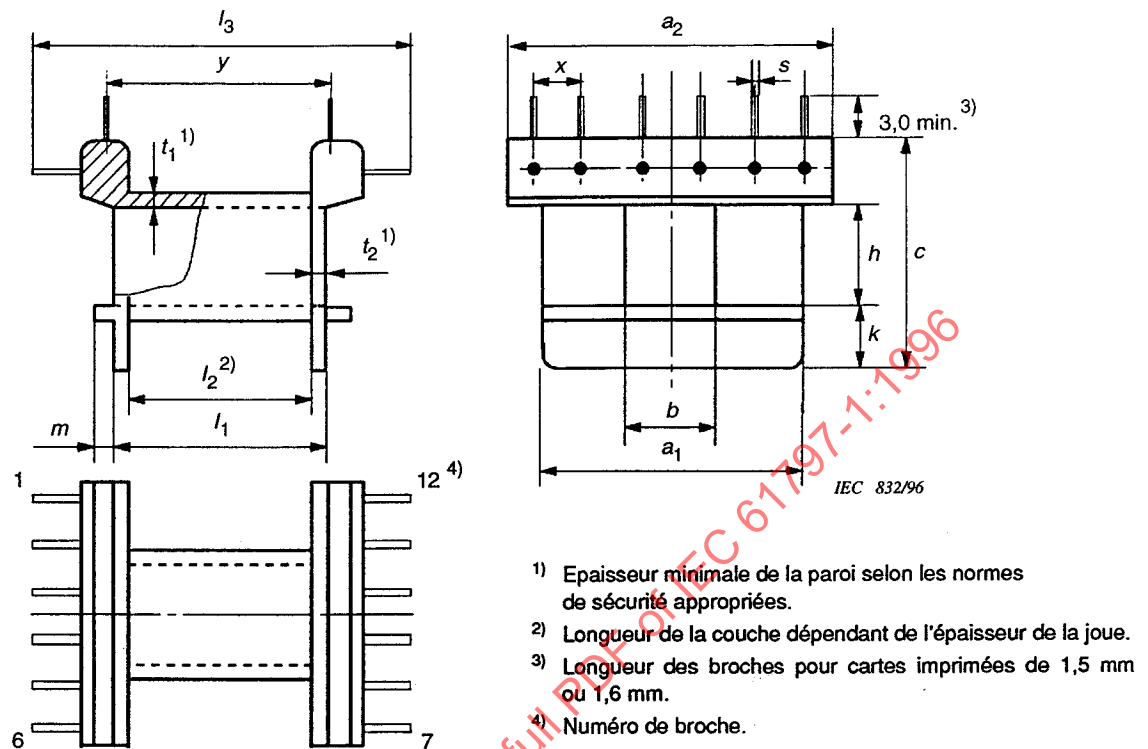
Figure 13 – Carcasses YM 1 pour montage sur carte à câblage imprimé, mode de montage à plat
