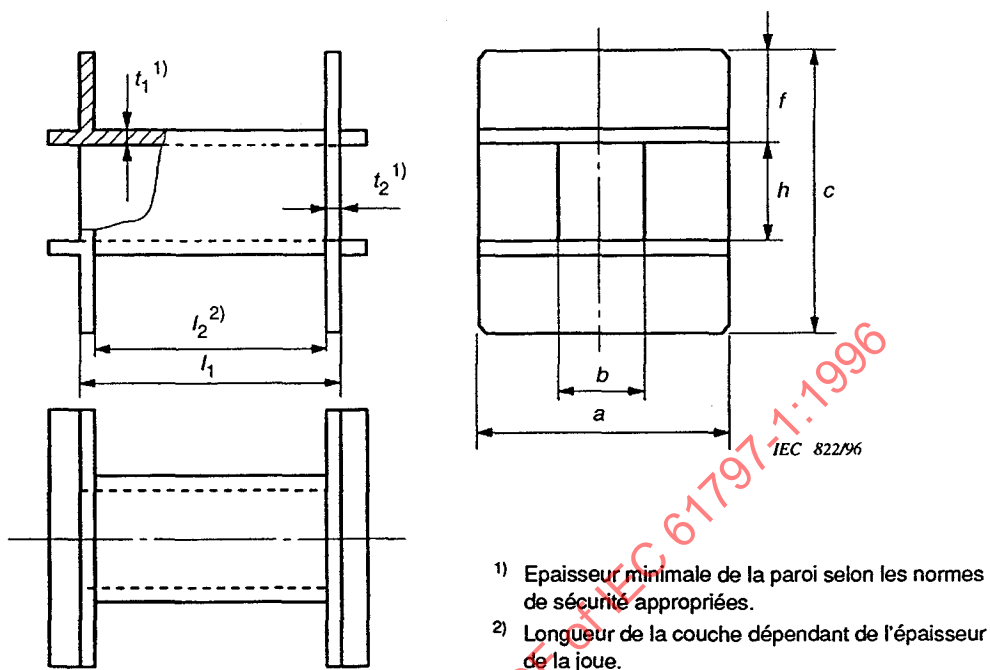
Figure 3 – Carcasses YUI 1 pour montage sur cornières et sur montants, version normalisée
