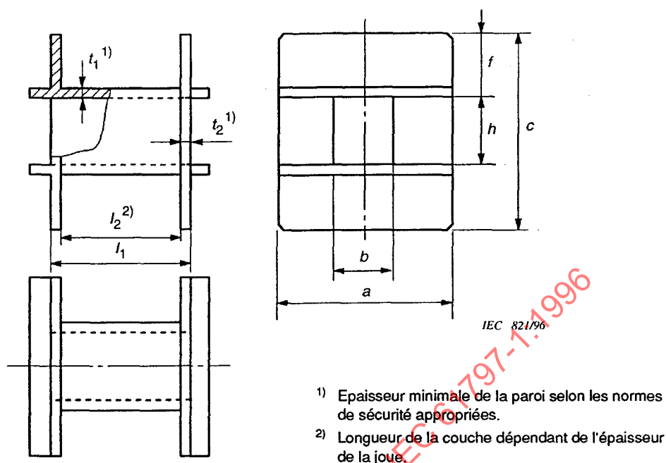
Figure 2 – Carcasses YEx 2 pour montage sur cornières et avec étrier U, version normalisée
